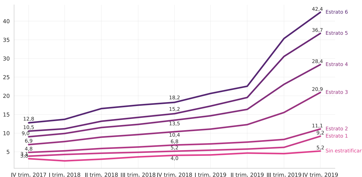
Gráfico 12. Velocidad de descarga promedio por estrato (Mbps)
