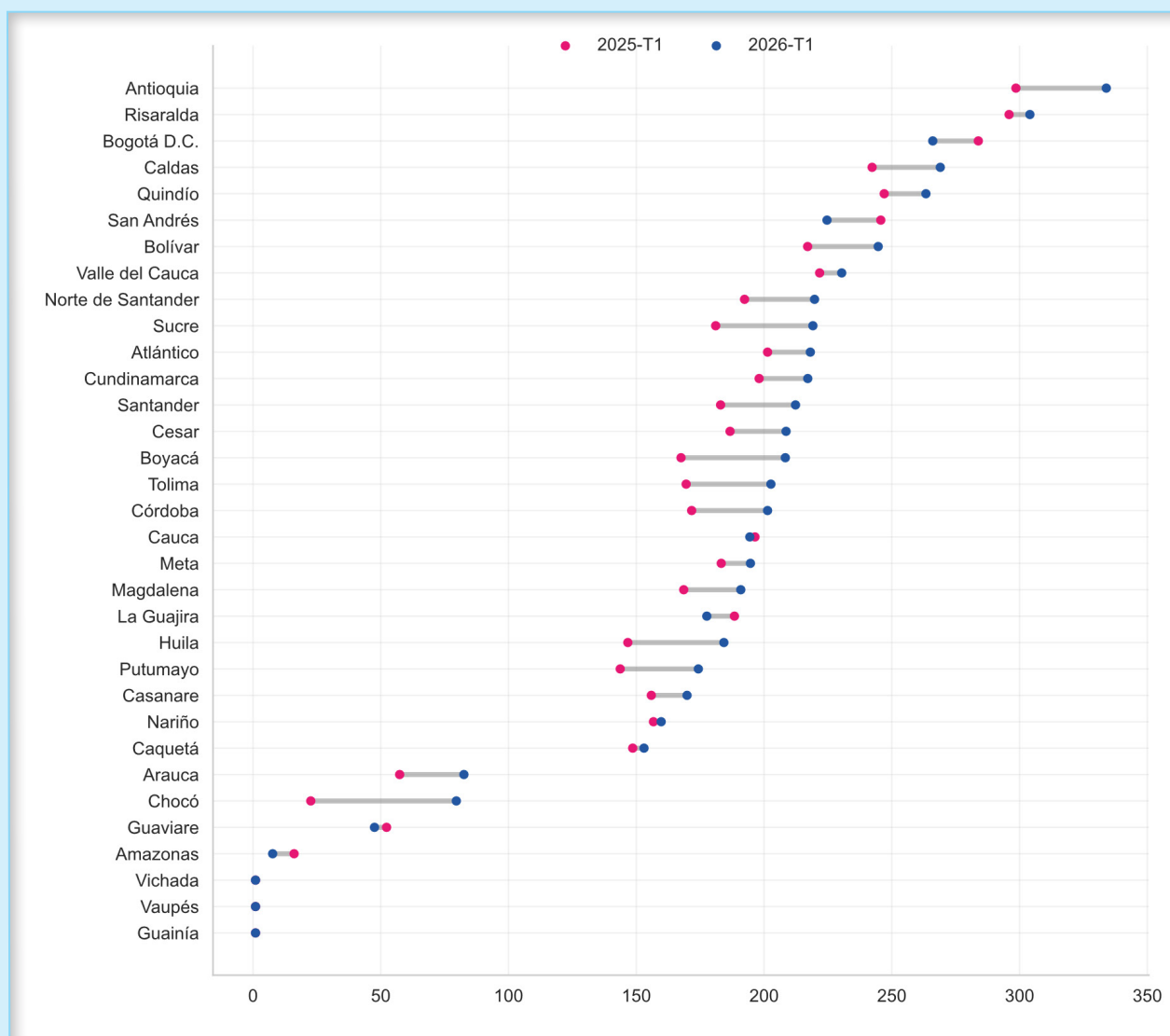
Gráfico 17. Velocidad de descarga promedio en el segmento residencial por departamento (Mbps)
