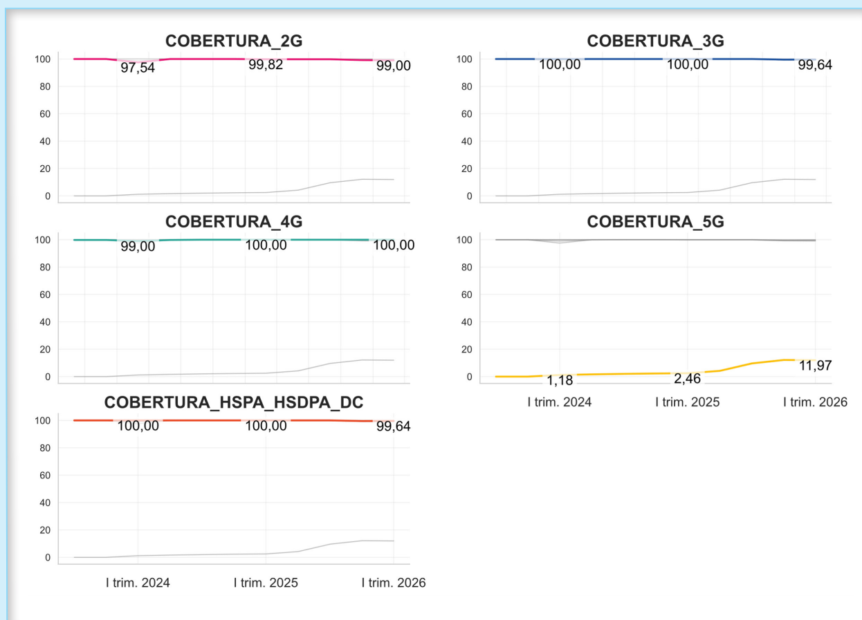
Gráfico 65. Porcentaje de municipios con cobertura por tecnología
